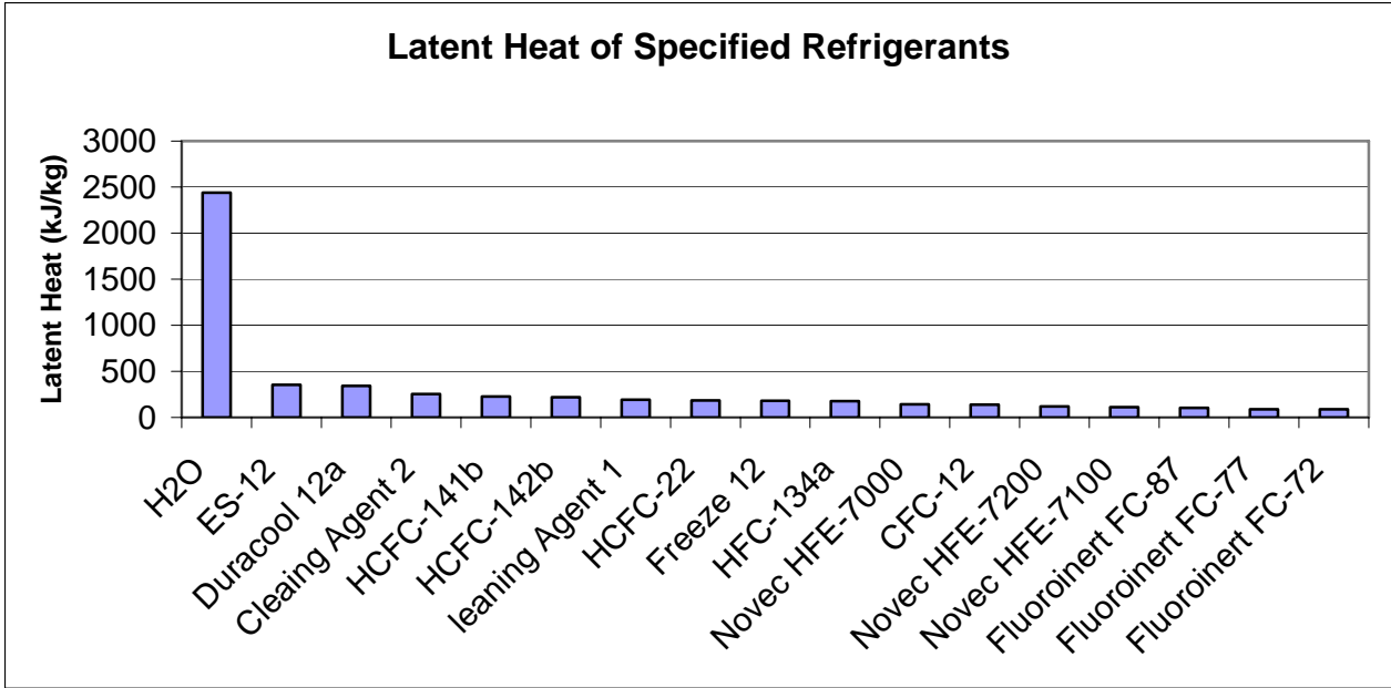
Fig. 3. Latent heat.
