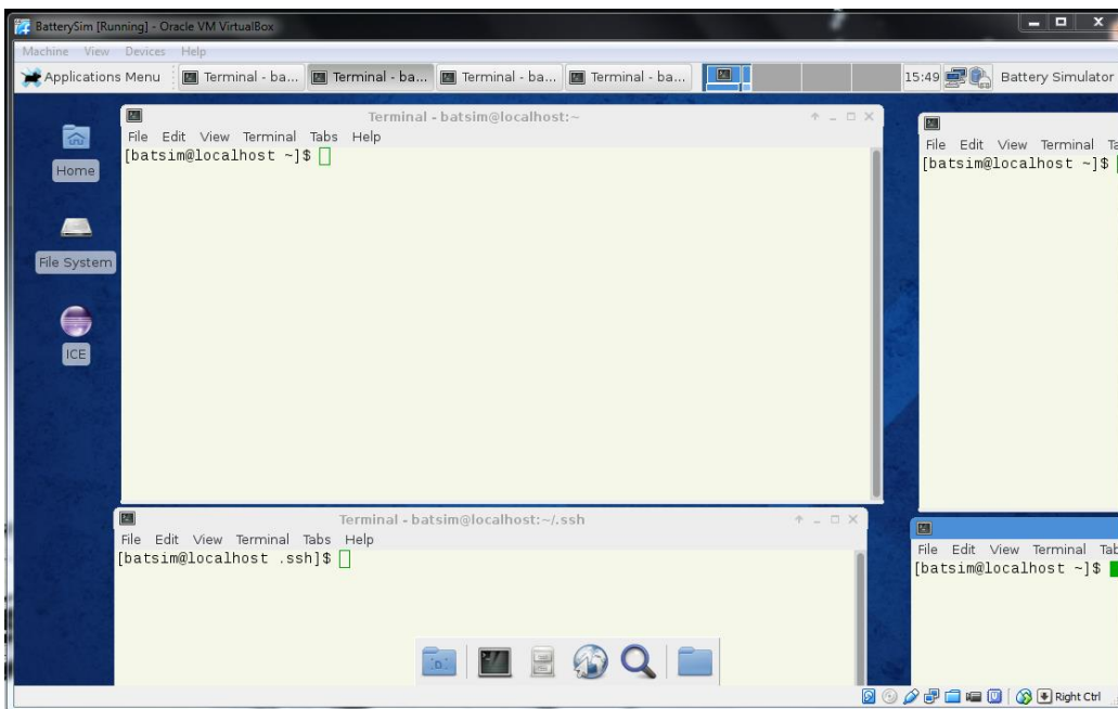
Fig. 16. BatterySim VM
